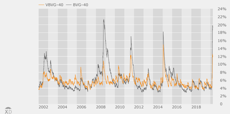
VBVG-40 vs BVG-40 Ex-post Volatilität 01.01.02–31.03.20
