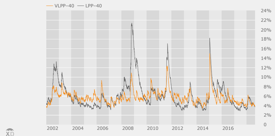
VLPP-40 vs LPP-40 Volatilité ex post 01.01.02-31.08.18
