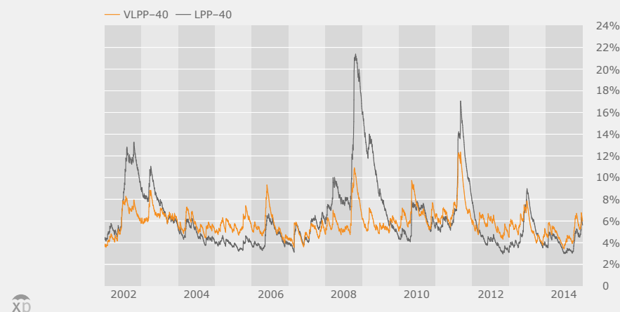
VLPP-40 vs LPP-40 Volatilité ex post 01.01.02–31.12.14
