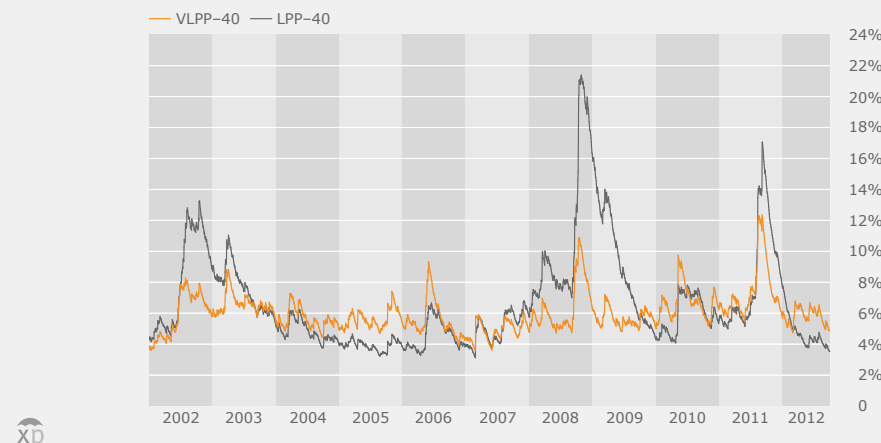
VLPP-40 vs LPP-40 Volatilité ex post 01.01.02-28.09.12
