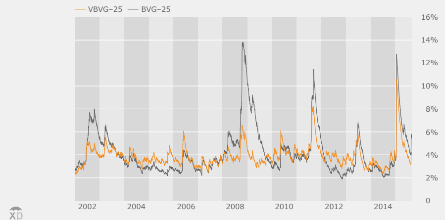
VBVG-25 vs BVG-25 Ex-post Volatilität 01.01.02–31.08.15
