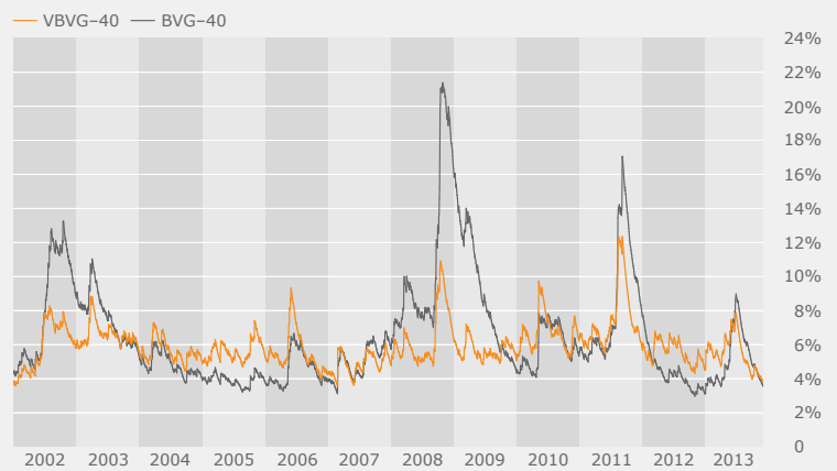
VBVG-40 vs BVG-40 Ex-post Volatilität 01.01.02–29.11.13
