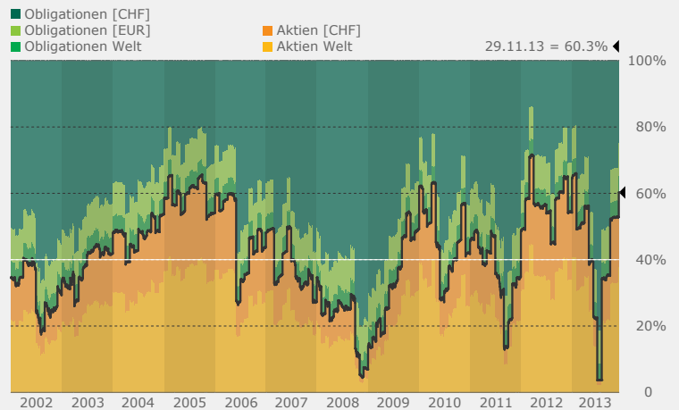
Fundo VBVG-40 Gewichtung Anlageklassen 01.01.02–29.11.13
